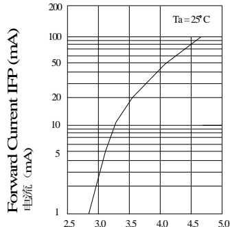
Forward Voltage (V) 电压 (V)
