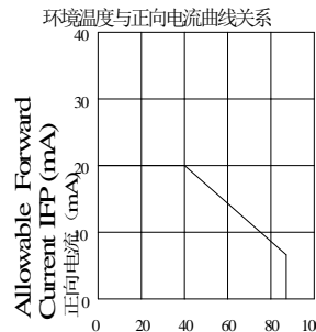
Ambient Temperature (°C) 环境温度 (°C)
