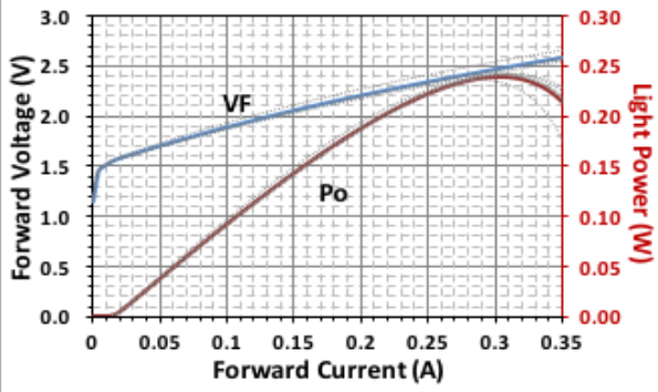
LIV Curve
